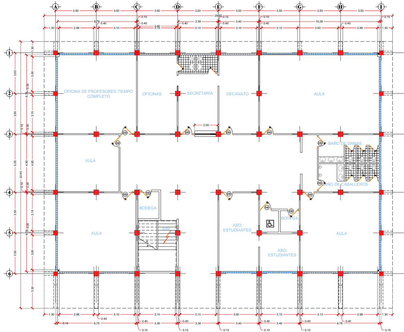
PLANO ARQUITECTÓNICA FACULTAD DE AGROPECUARIA PLANTA BAJA
