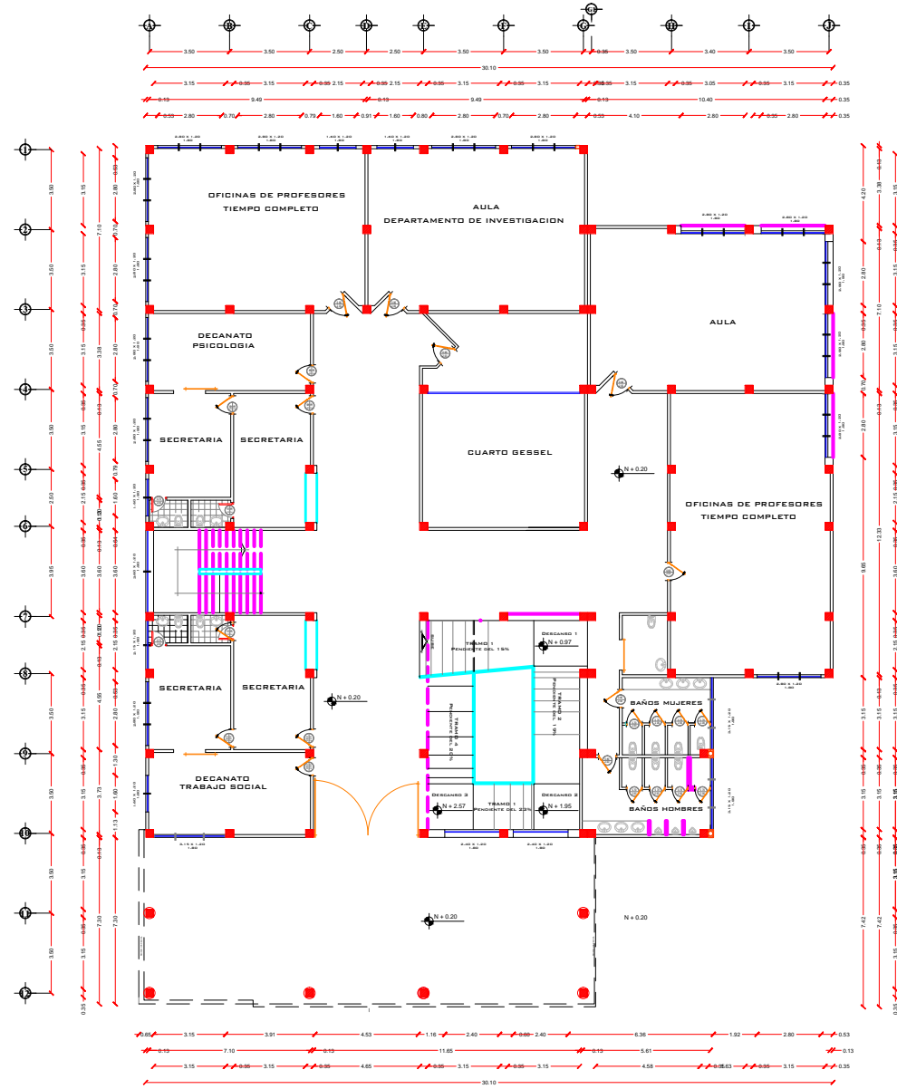
PLANTA ARQUITECTÓNICA FACULTAD DE TRABAJO SOCIAL PLANTA BAJA 1:300
